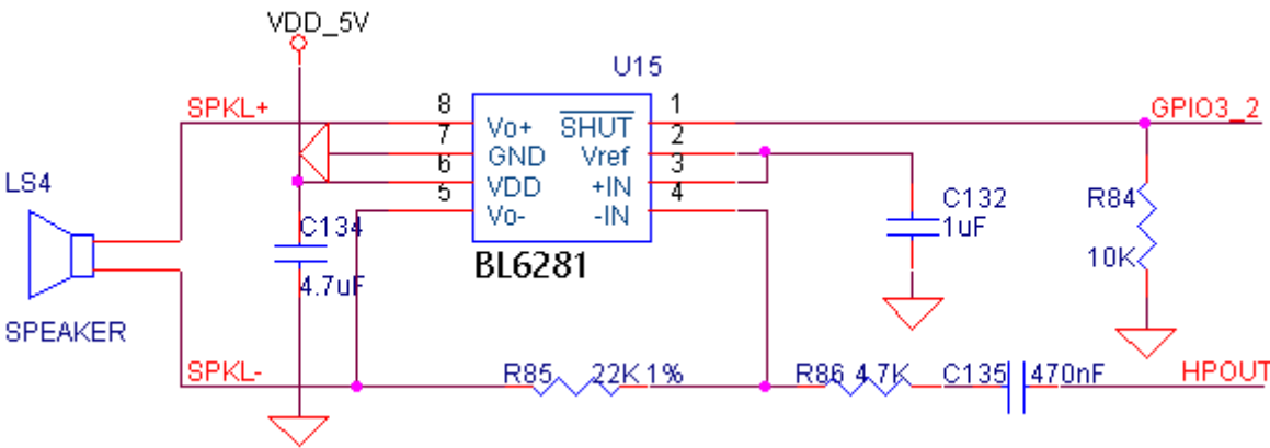
图21 功放电路图
