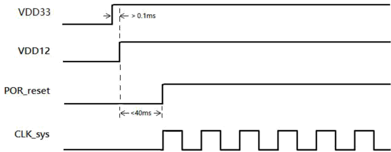
图7 上电时序图
