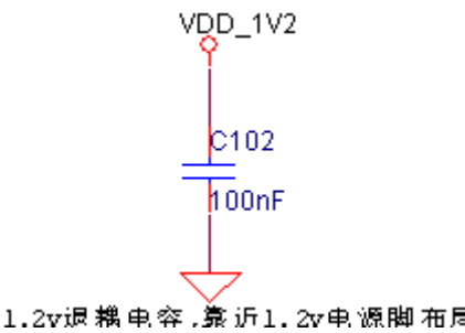
图14 CPU 1.2V滤波电路图
