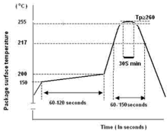
图24 CI1122 SMT焊接温度曲线
