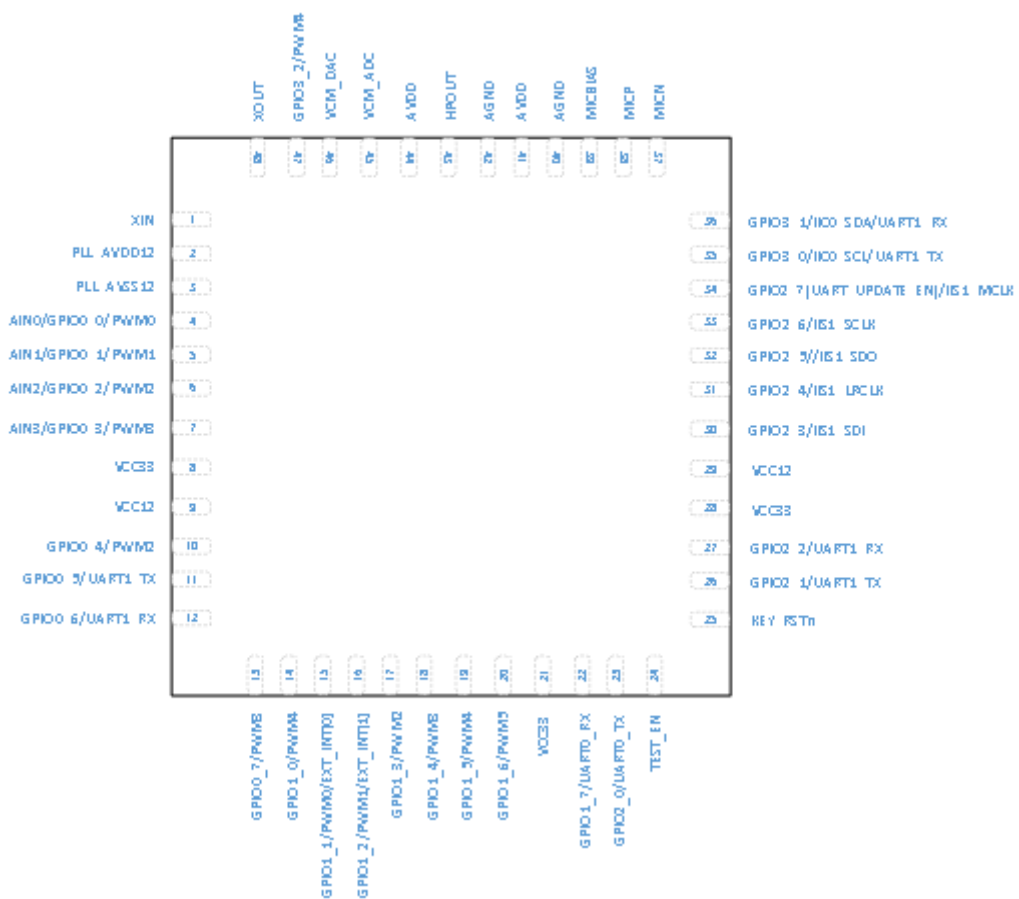
图2 CI1122芯片引脚图
