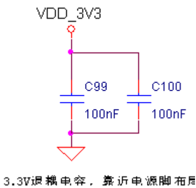
图13 CPU 3.3V滤波电路图
