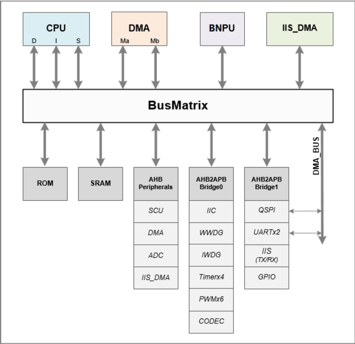
图4 CI1122系统架构
