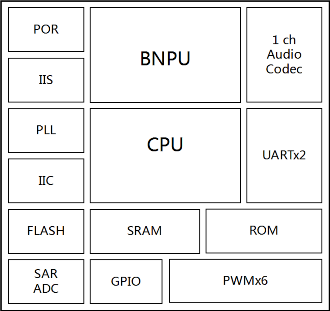
图3 CI1122系统框图
