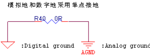
图17 模拟地和数字地的分割
