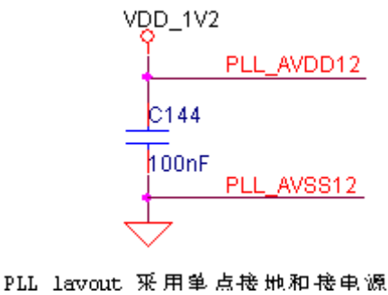
图15 CPU PLL电源滤波电路图
