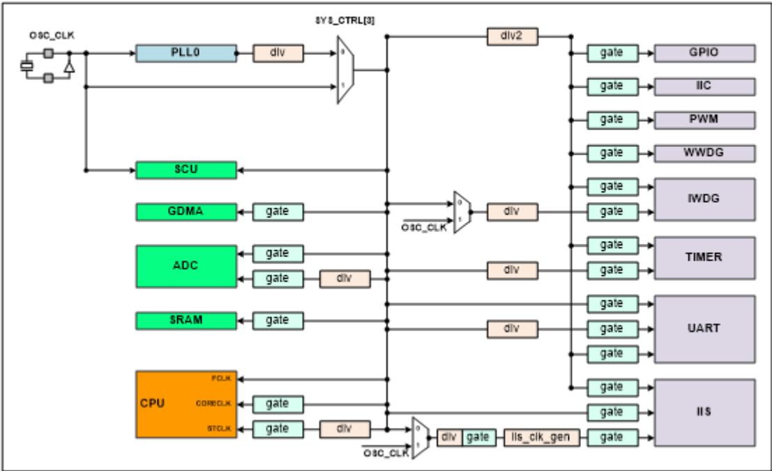
图6 时钟结构
