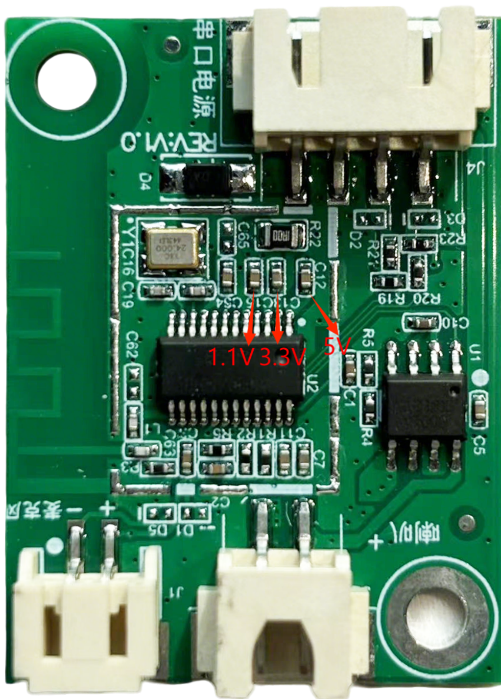
图17 模块测试点分布图
