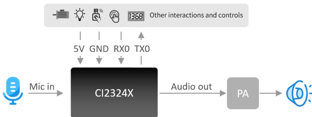
图1 模块框图
