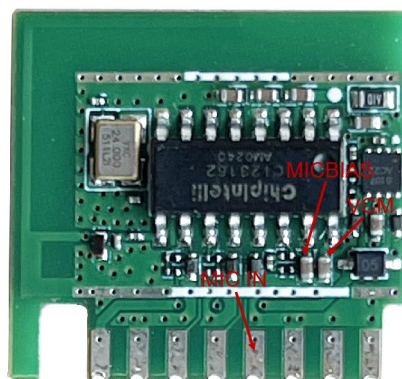
图 16 模块麦克风信号测试点
