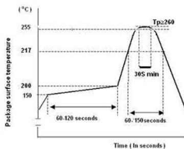
图 18 模组贴装炉温曲线
