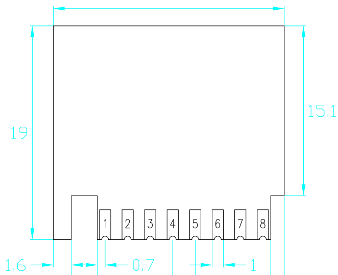
图 5 模块尺寸图
