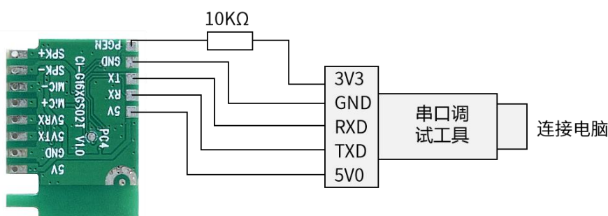
图 11 模块和 USB 转串口工具连接图
