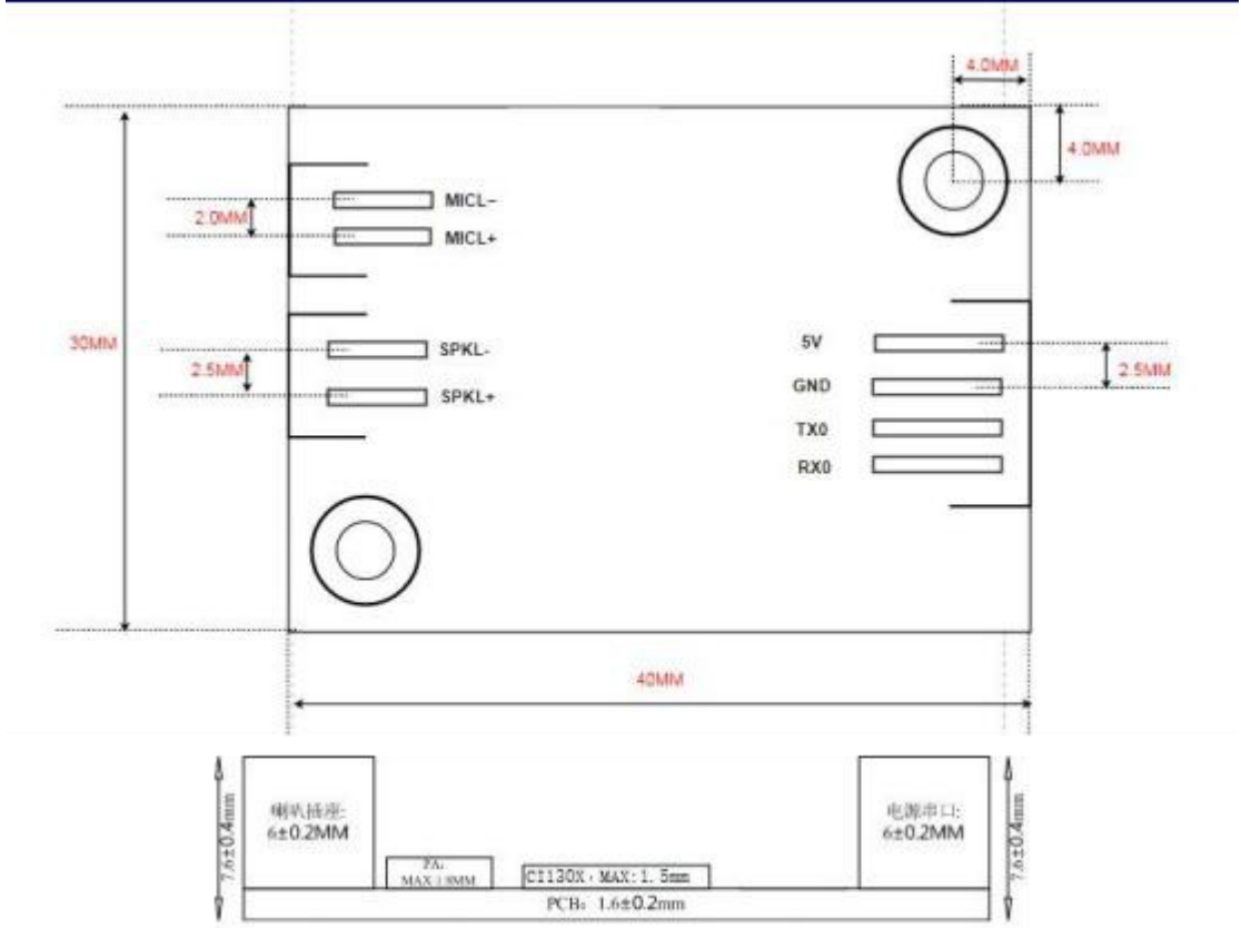
图 5 模块尺寸图
