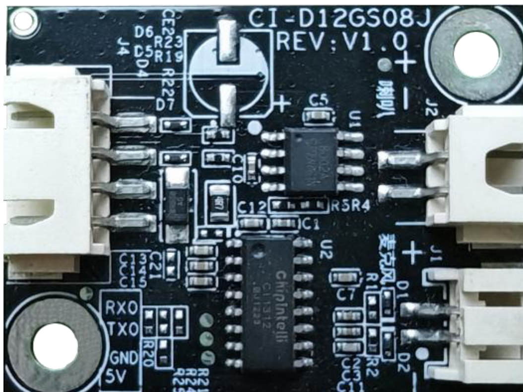
图 4 模块实物图
