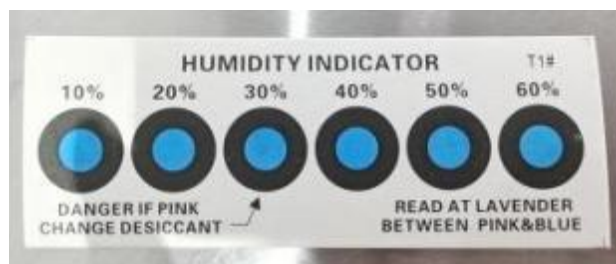
图 17 湿度指示卡
