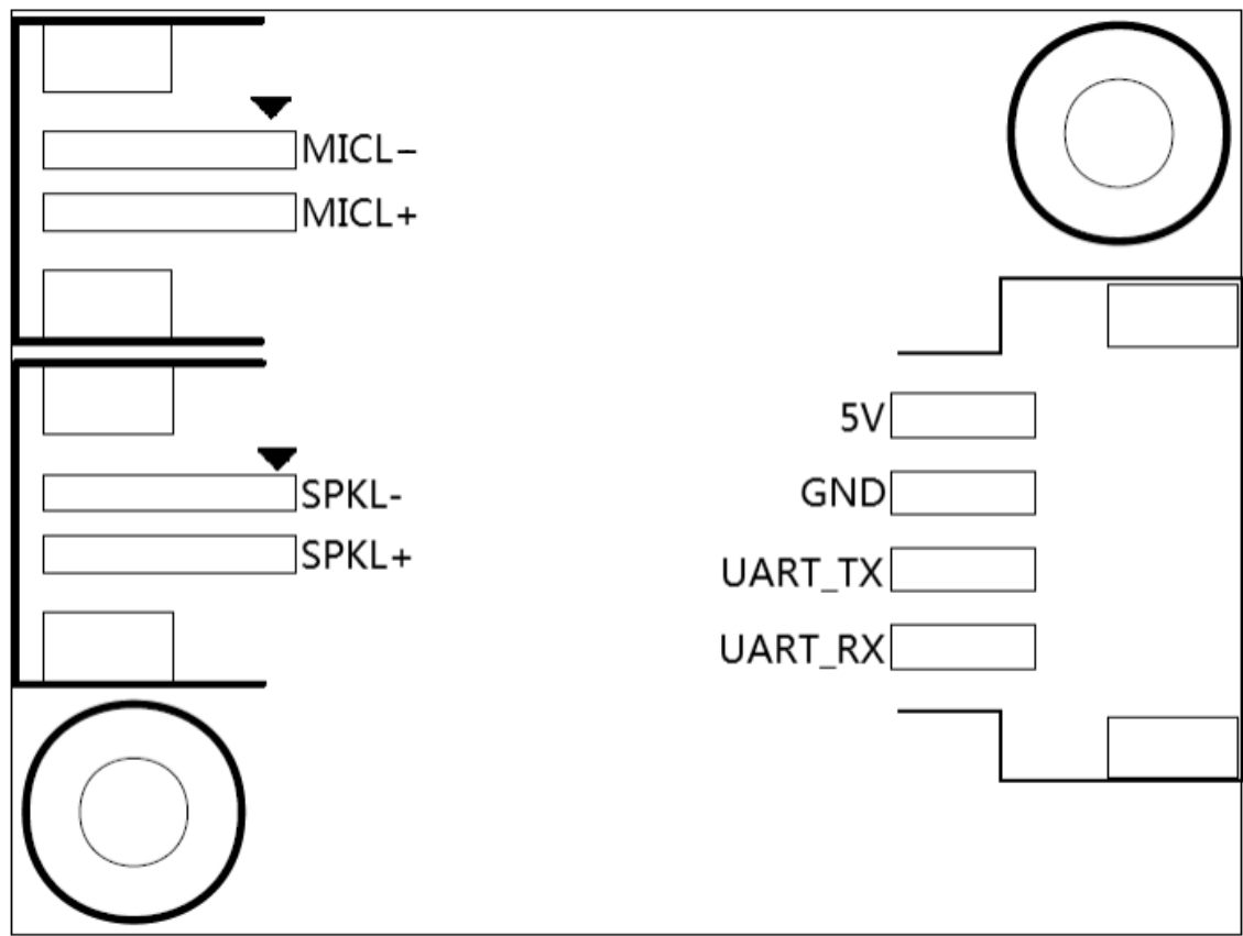
图6 模块引脚图
