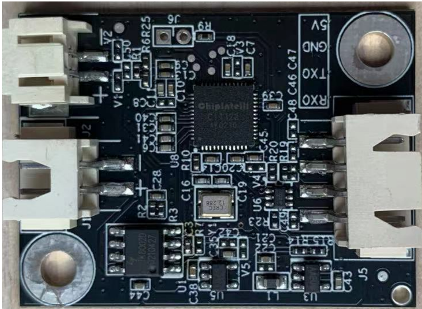
模块实物图
