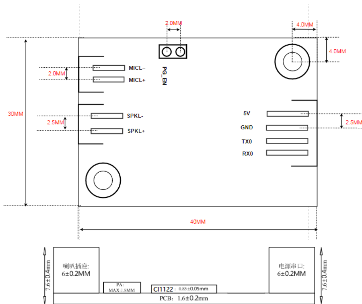
图5 模块尺寸图
