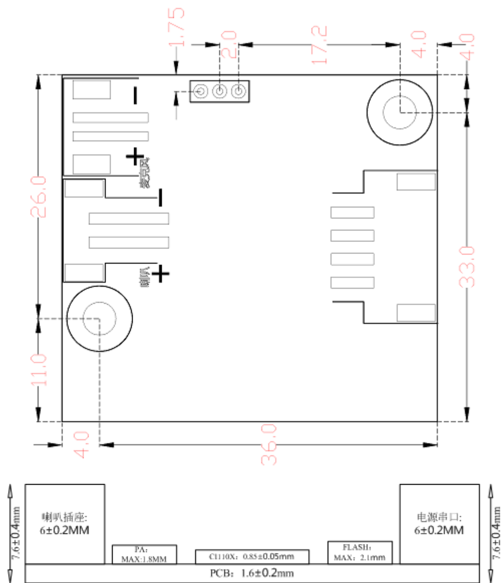
图5 模块尺寸图
