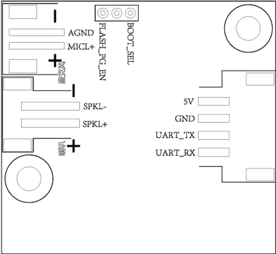
图6 模块引脚图
