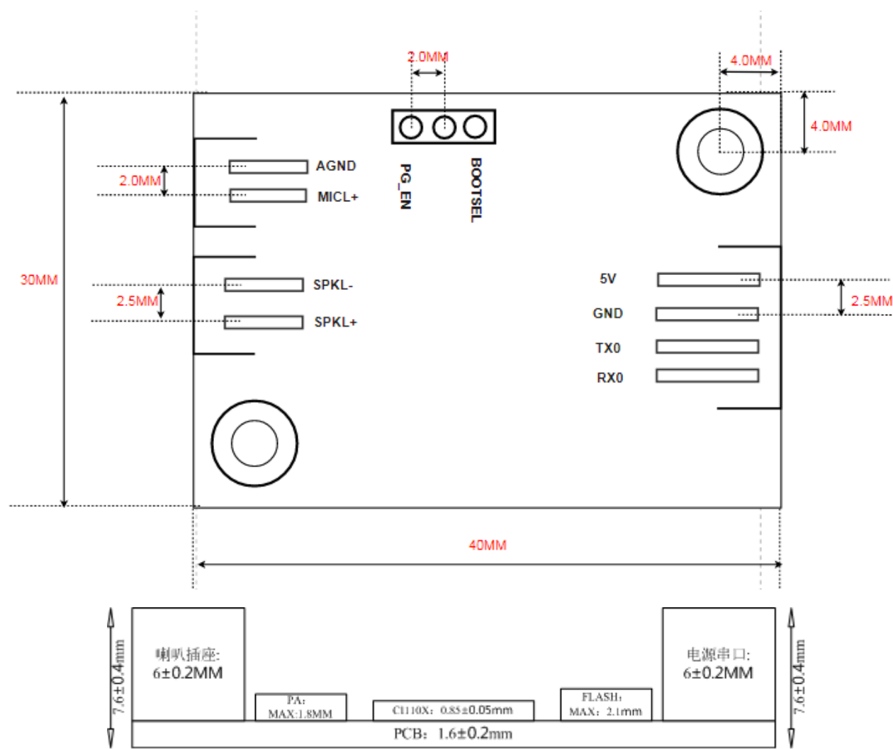
图5 模块尺寸图
