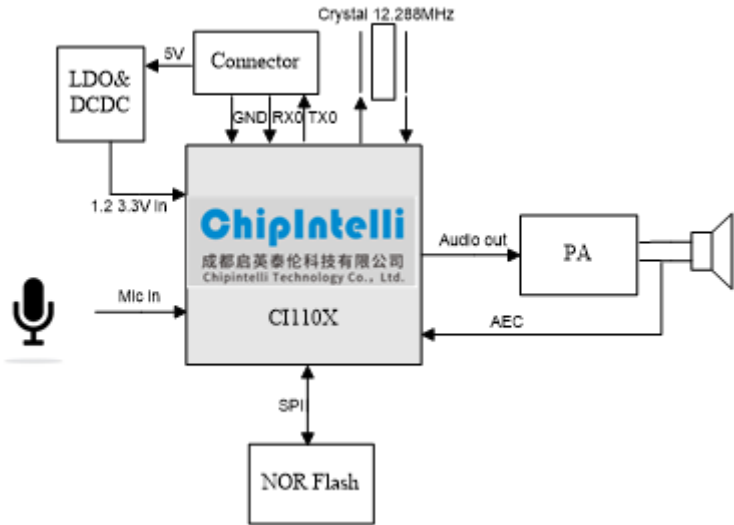
图1 模块框图
