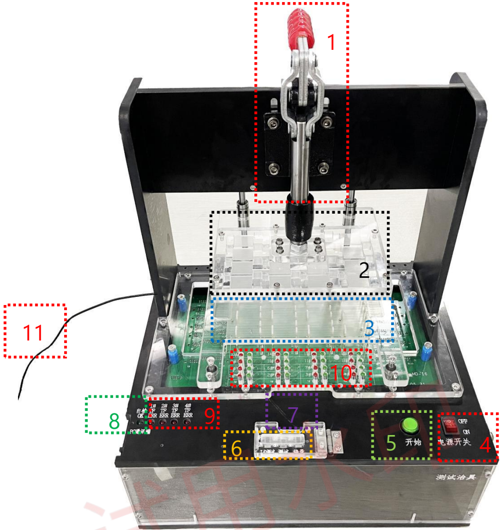
图 1-1 产测治具外部组件图（对应表 1-1）
